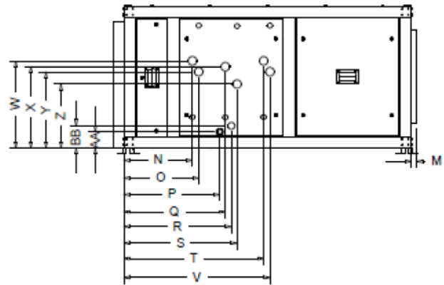
UNIDAD HORIZONTAL PARED SENCILLA O DOBLE DE 024 A 120
