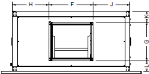
UNIDAD HORIZONTAL PARED SENCILLA O DOBLE DE 024 A 120
